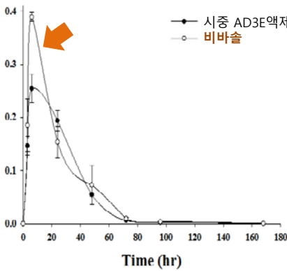
비타민 A
