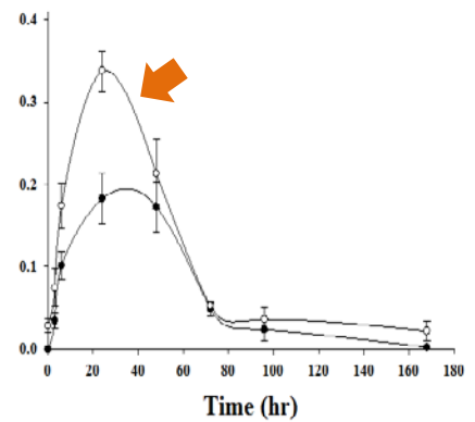
비타민 E(OAc+OH)
