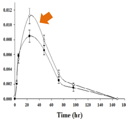
비타민 D3
